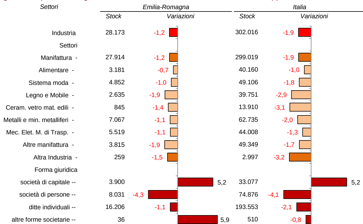
Fig. 2.12.9. Imprese attive artigiane dell'industria in senso stretto e tassi di variazione tendenziali (1). 3° trimestre 2018
