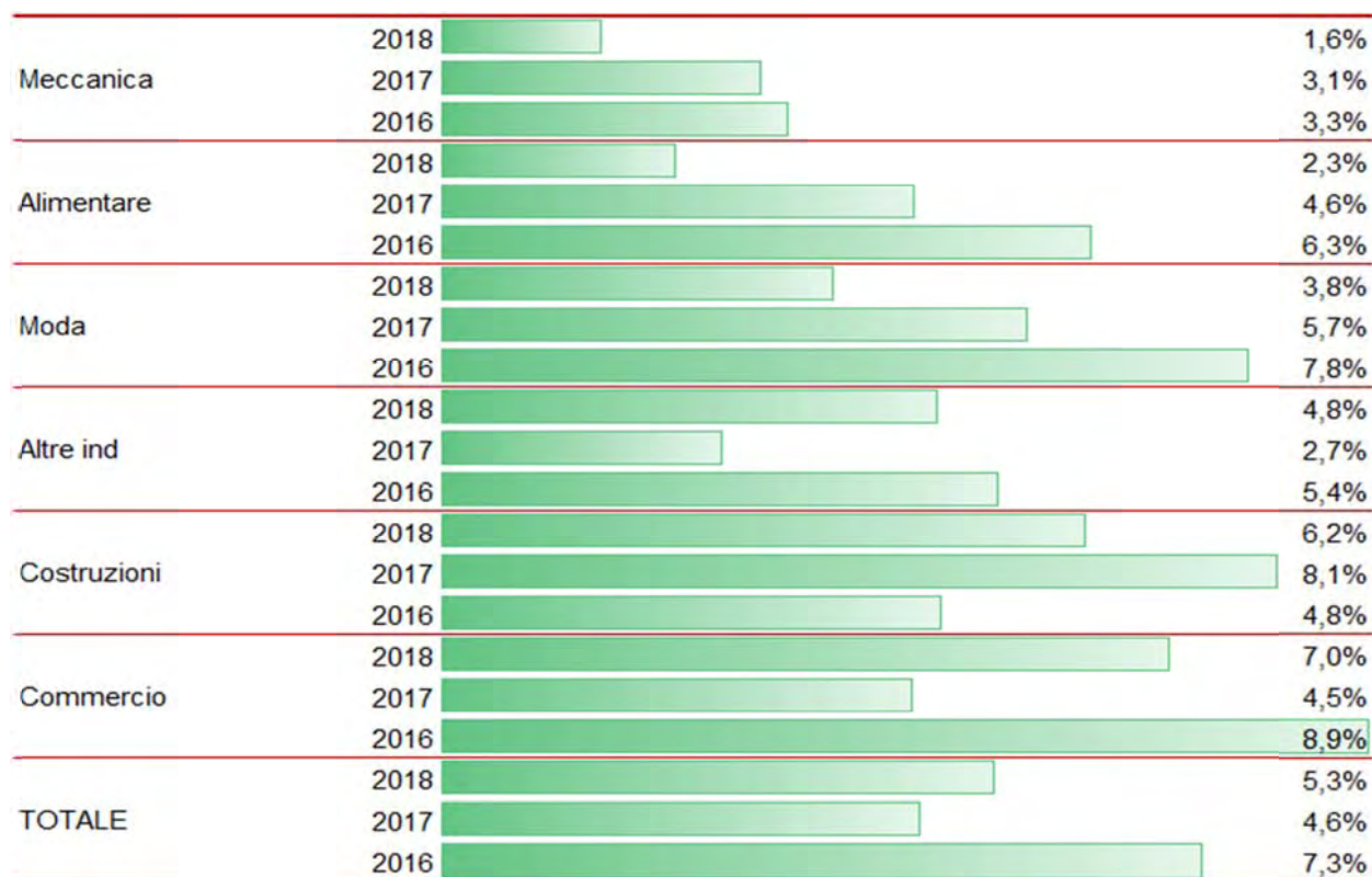
Fig. 2.11.9. Incidenza percentuale delle imprese che non sono sempre state in grado di far fronte ai propri impegni nei primi 6 mesi dell'anno. Anni 2018, 2017 e 2016.
