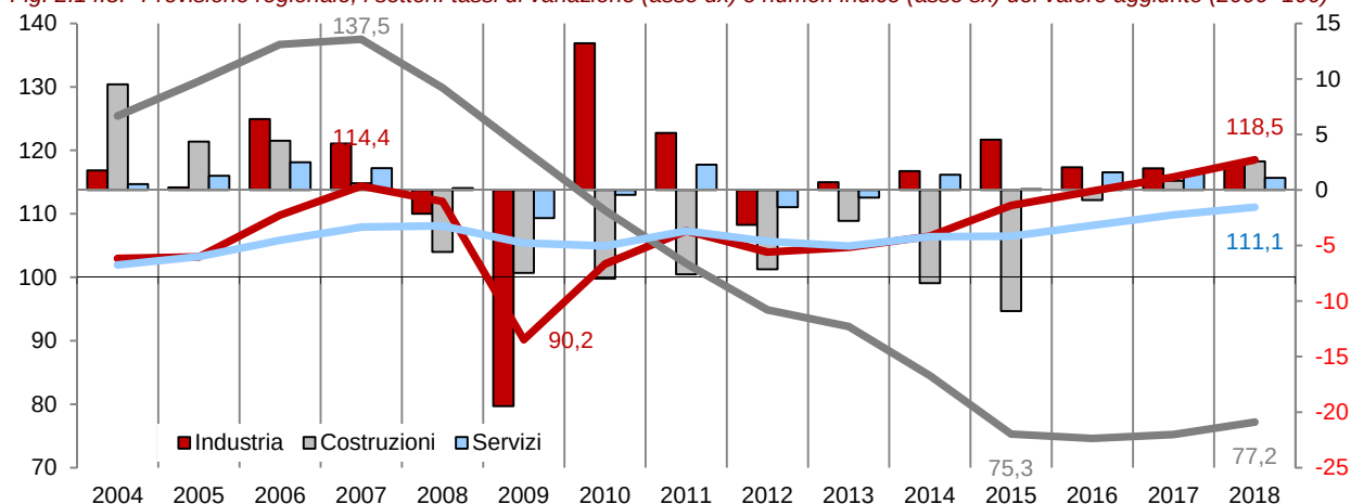
Fig. 2.14.8. Previsione regionale, i settori: tassi di variazione (asse dx) e numeri indice (asse sx) del valore aggiunto (2000=100)
