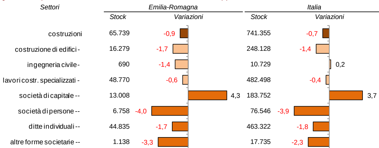
Fig. 2.6.5. Imprese attive delle costruzioni e tassi di variazione tendenziali (1). 3° trimestre 2018
